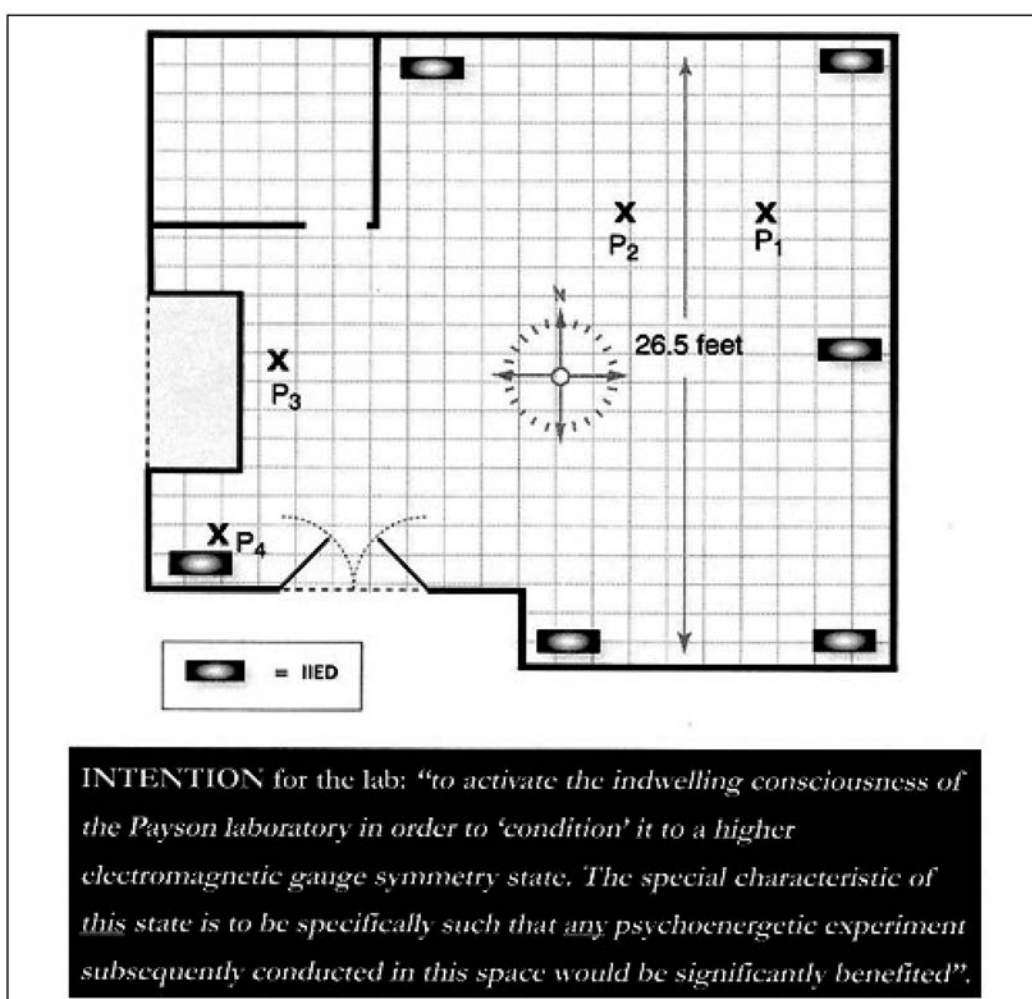
圖二、特定意念印記裝置IIED 安置於實驗室中遂行 意識→能量→水的酸鹼pH1 值變化實驗 17
