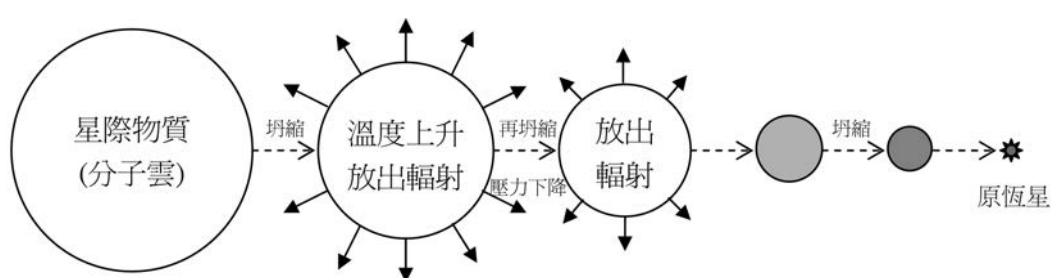
圖 1. 星際物質收縮放出射形成原恆星之示意圖 11
