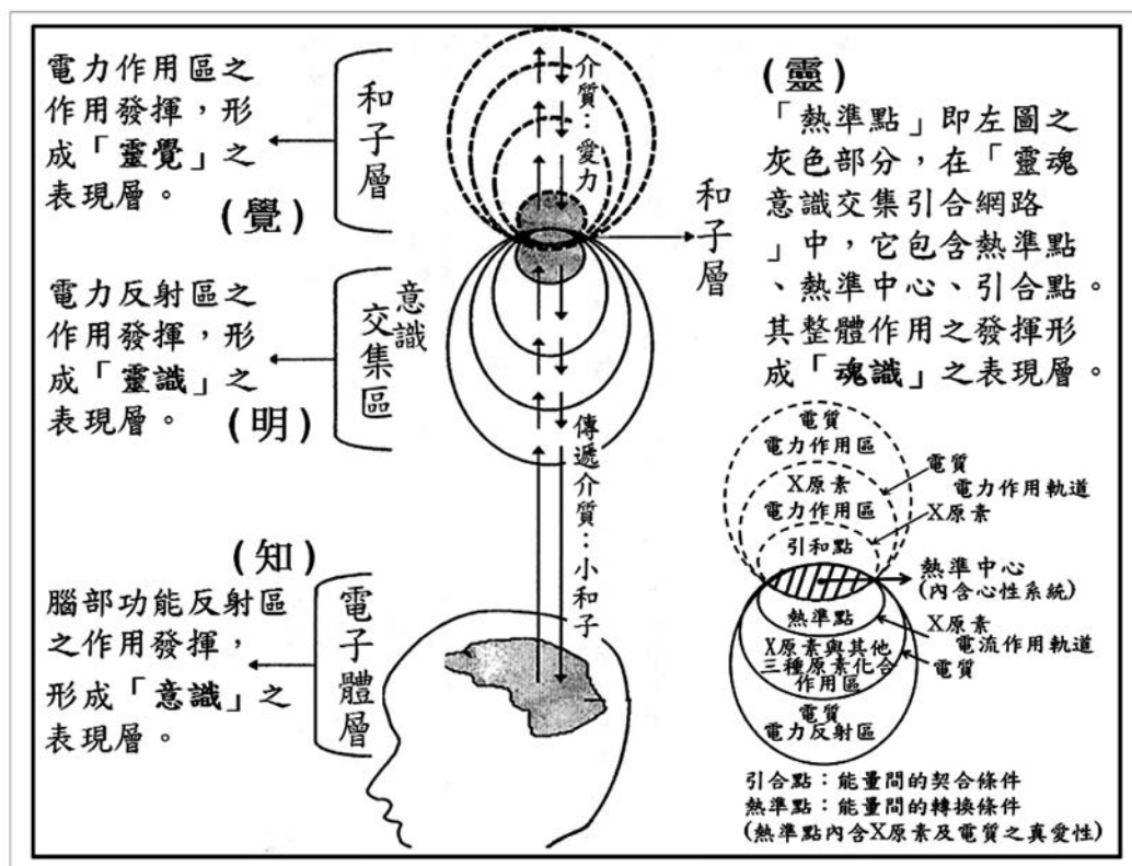
圖六、人類「靈魂意識交集引合網路」（虛實橢圓線圈）與「四大意識層」之運作關係圖（來回箭頭表示訊息傳遞；實線表示有形個體之訊息電流軌道，虛線表示無形電力軌道；實與虛四大軌道由外向內分別相應於和子的 O^{\circ} 精華、 H^{\circ} 精華、電質、X原素電流（磁場）與電力（電場）作用軌道；實與虛四大軌道之間分別相應於電力反射區與電力作用區；灰色部分統稱「熱準點」為X原素的作用範圍，經放大置於圖中右下角，又可細分為引合點、熱準中心、熱準點） 27
