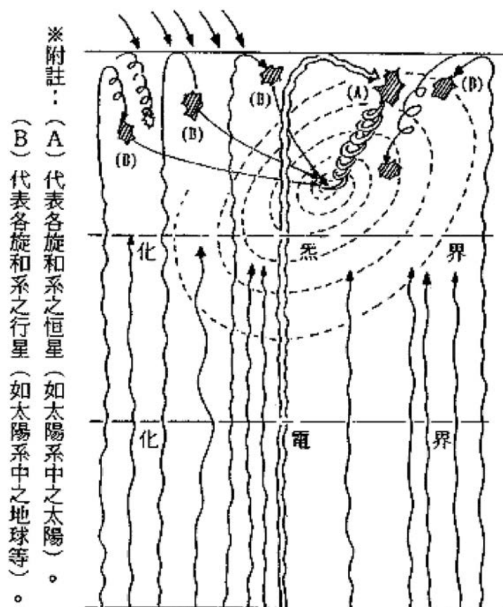
圖 2. 旋和系形成示意圖 25
