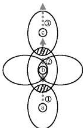
圖 3. 氧化原理示意圖
