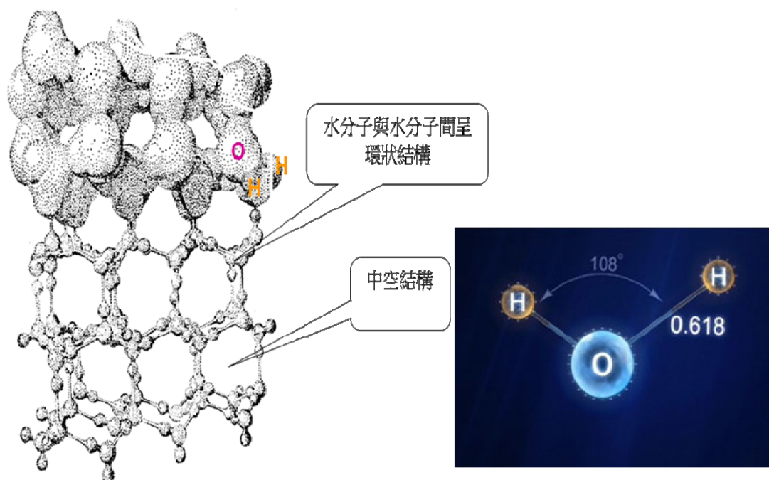
圖二、水分子的環狀中空結構與電雙極磁石特性 (化學鍵角 108 度、鍵長呈黃金比例 0.618) 9
